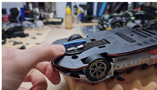
5.1 Die Metallfeder muss den Schwingarm hochdrücken
